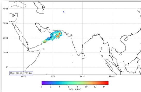
TROPOMI 24.11.25
