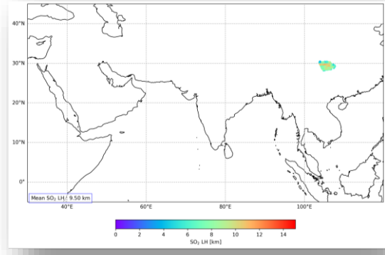
TROPOMI 25.11.25
